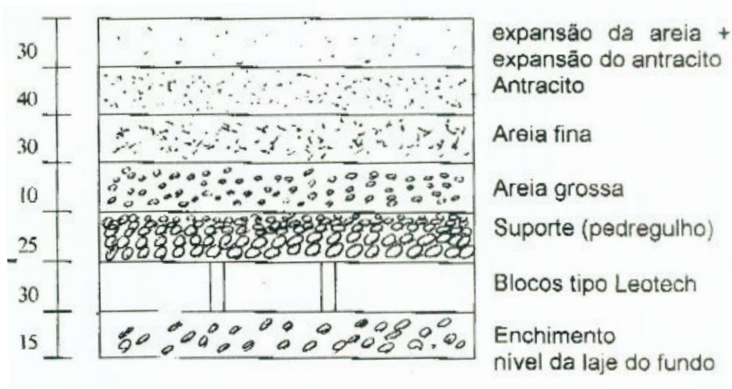
Desenho 03 – Perfil Ilustrativo do Filtro (imagem sem escala)
