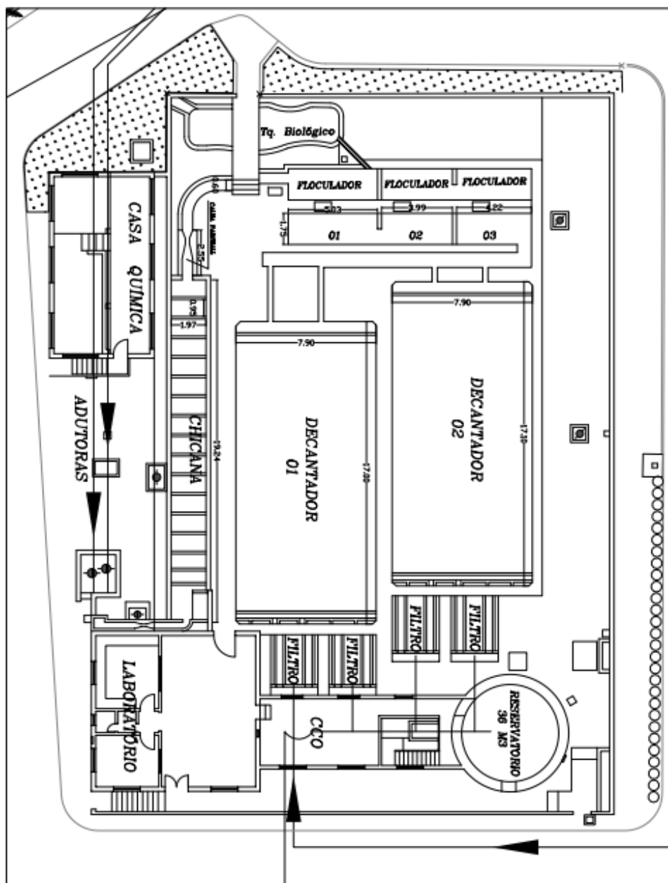
Figura 2 - Vista da Concepção Original da ETA (em processo de readequação) com vista dos filtros
