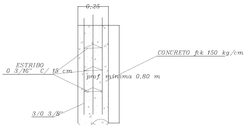
Imagem 2: Detalhamento ferragem Brocas
