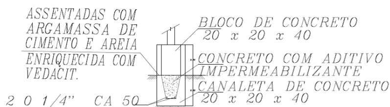
Imagem 3: Detalhamento viga baldrame
