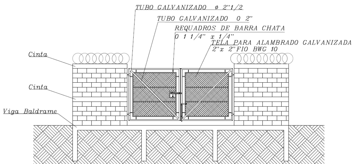
Imagem 4: Modelo muro + portão
